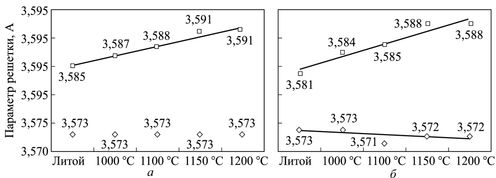
Рис. 4. Зависимость параметров решеток фаз сплавов от температуры отжига: а – ВКНА-4У; б – ВКНА-1В: ◇ – ВКНА-4У; □ – ВКНА-1В
