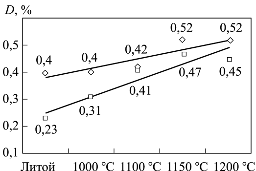
Рис. 5. Зависимость несоответствия параметров кристаллических решеток \gamma и \gamma' -фаз от температуры отжига: ◇ – ВКНА-4У; □ – ВКНА-1В
