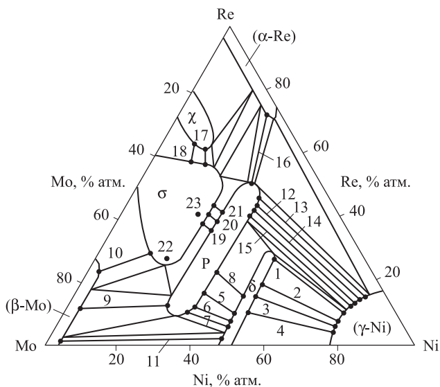
Рис. 8. Изотермическое сечение трехкомпонентной системы Ni–Re–Mo при температуре 1375 К (1102 °С) [18]
