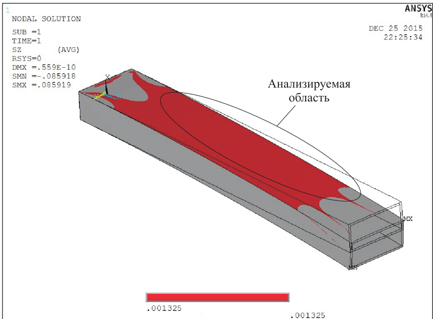
Рис. 3. Расчет прямого участка волновода в ANSYS:
