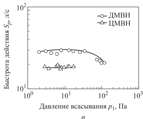
Рис. 5 (окончание). Сравнение результатов расчета по разработанной математической модели с результатами эксперимента:
