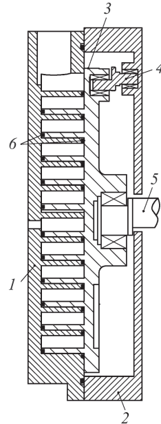
Рис. 6. Схема НВСп:
